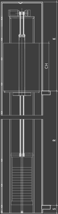
Hoistway Elevation
