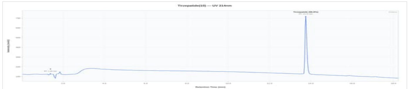
AEO-TRZ 10 - AEON-TR10-C1726: UV Chromatogram
