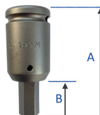
Douille Porte Embout avec embouts hexagonaux interchangeables
