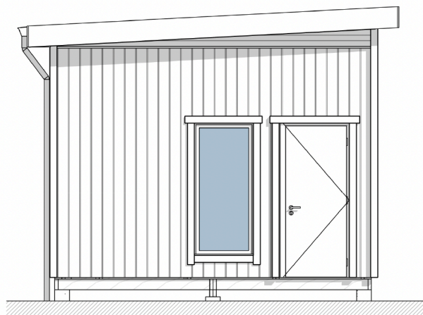
1 FASAD GAVEL 1 1 : 50
