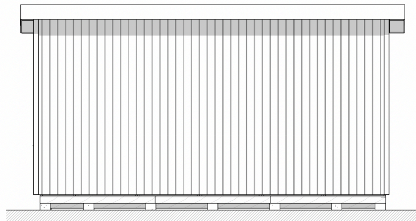
3 FASAD LÅNGSIDA 1 1 : 50
