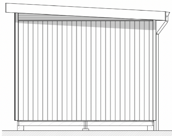
2 FASAD GAVEL 2 1 : 50
