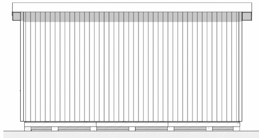
3 FASAD LÅNGSIDA 1 1 : 50
