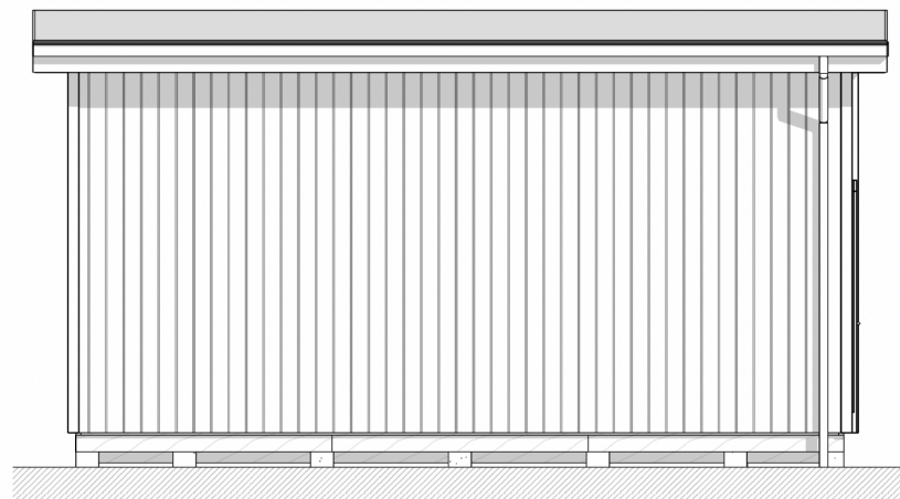
4 FASAD LÅNGSIDA 2 1 : 50
